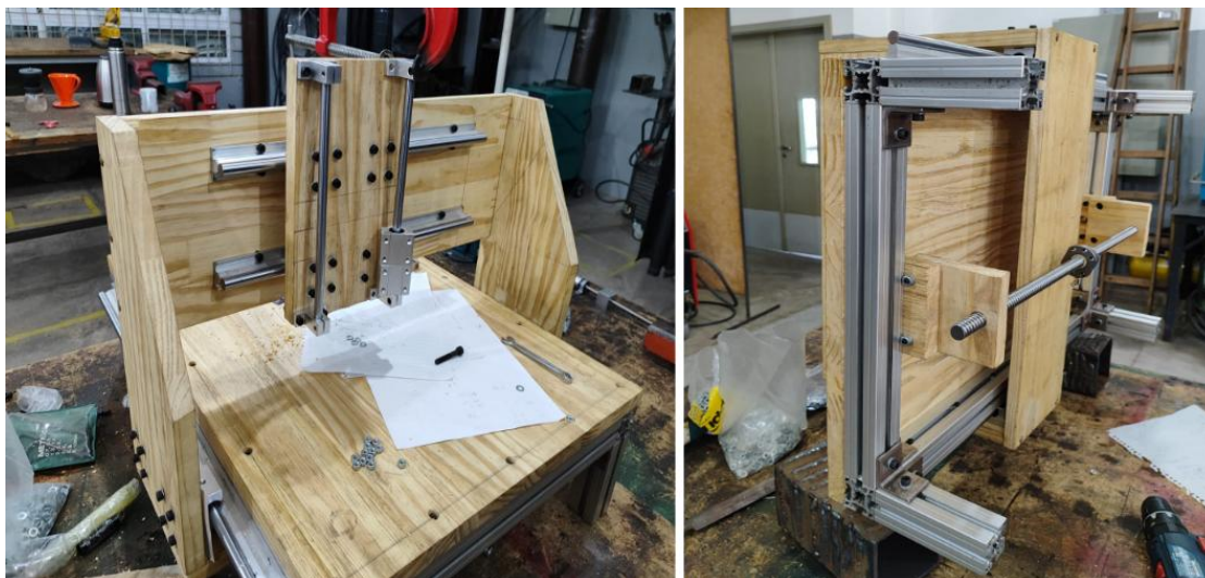
Figura 5 – (a) guias lineares do eixo z; (b) fuso de movimentação do eixo y
